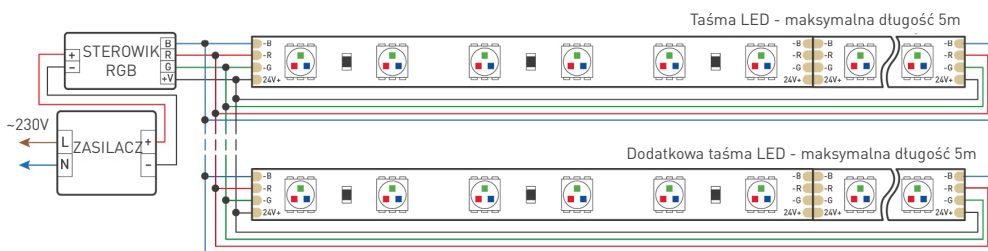
Schemat 2. Podłączenie kilku taśm LED z zasilaniem z obu stron. Zalecany schemat podłączenia w celu zapewnienia równomiernego natężenia oświetlenia na całej długości taśmy LED.
